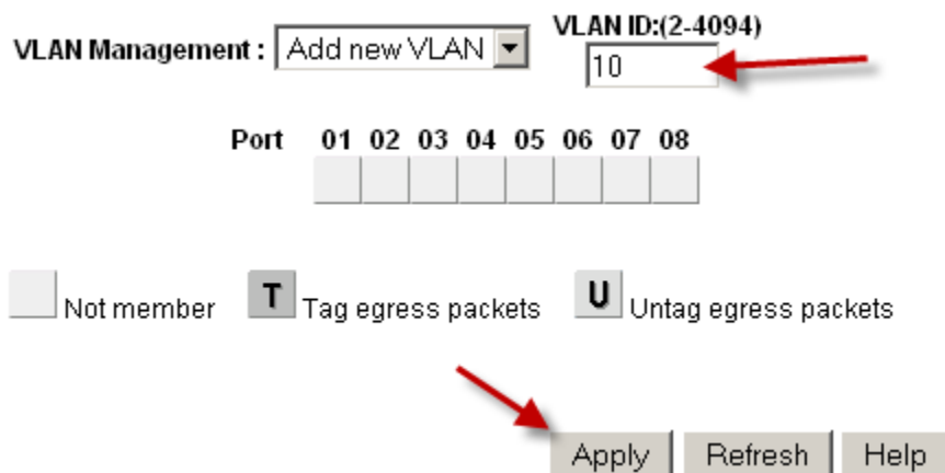
Fig. 105: Add VLAN 10
